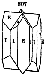
Staurolite.
